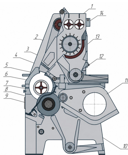
Рисунок 1. Линтер 5-LP (схема заимствована из паспорта пильного волокноотделителя 4ДП-130 [11] и переработана авторами): 1 — питатель типа КПП; 2 — семяобразующий лоток; 3 — резиновая заслонка, предотвращающая обратный выход семян из рабочей камеры; 4 — рабочая (семенная) камера; 5 — распылитель; 6 — пильный цилиндр; 7 — воздушная камера; 8 — конвейер улюка; 9 — конвейер отходов; 10 — электропереключатель; 11 — основание.
