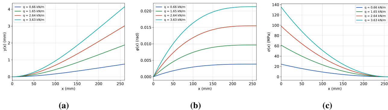
Рисунок 4. Стенка из стали 3, h = 5,5 мм, при q = 0,66–3,63 кН/м: (а) прогиб, (б) угол поворота, (в) напряжение.
