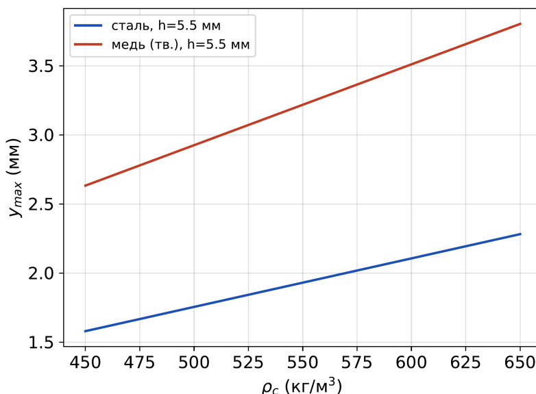
Рисунок 6. Калибровочная зависимость по формуле (11), h = 5,5 мм, n = 775 об/мин.
