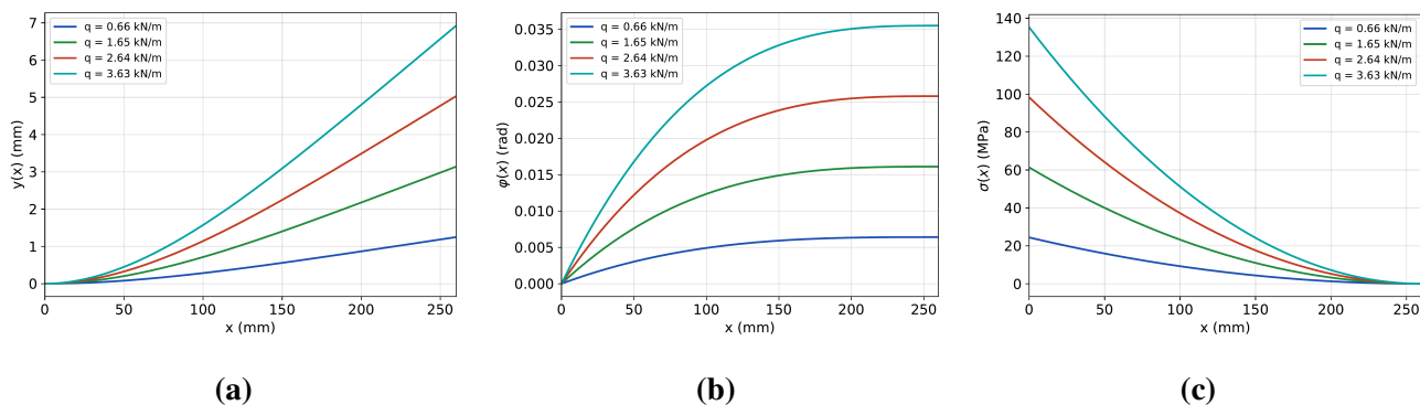
Рисунок 5. Стенка из твёрдой (наклёпанной) меди, h = 5,5 мм, при q = 0,66–3,63 кН/м: (а) прогиб, (б) угол поворота, (в) напряжение.
