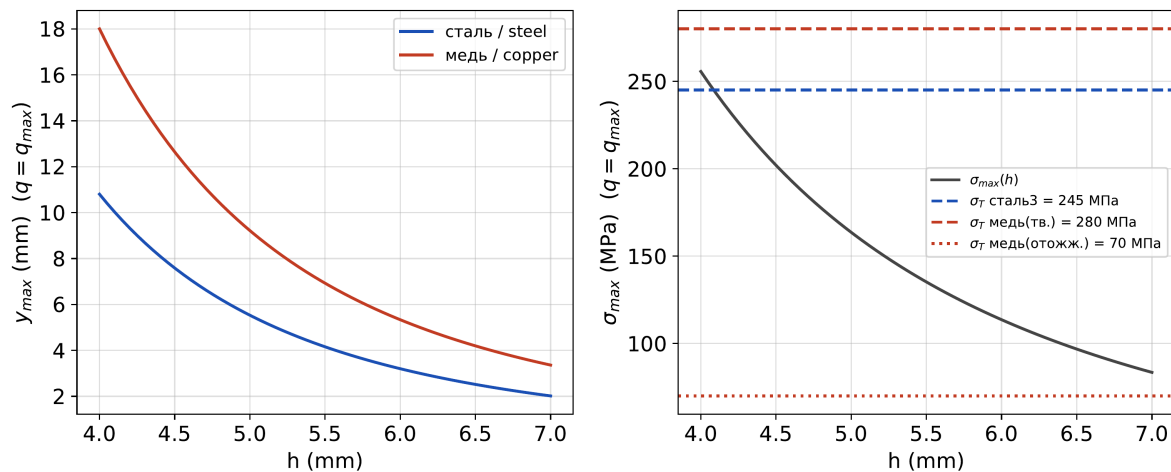
Рисунок 3. Зависимость максимального прогиба (слева) и максимального напряжения (справа) от толщины стенки при q = q_{\max} = 3,63 кН/м. Горизонтальные линии показывают пределы текучести стали 3, твёрдой и отожжённой меди.
