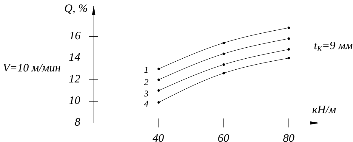
Рисунок 3. График удаленной влаги из кожевенного полуфабриката от сочетания пар отжимных валов, давления прижима P=40;60;80 кН/м и скорости пропуска V=10 м/мин
