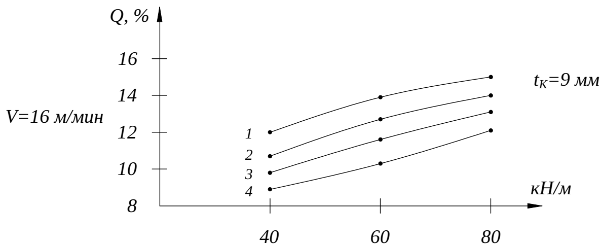
Рисунок 4. График удаленной влаги из кожевенного полуфабриката от сочетания пар отжимных валов, давления прижима P=40; 60; 80 кН/м и скорости пропускa V=16 м/мин
