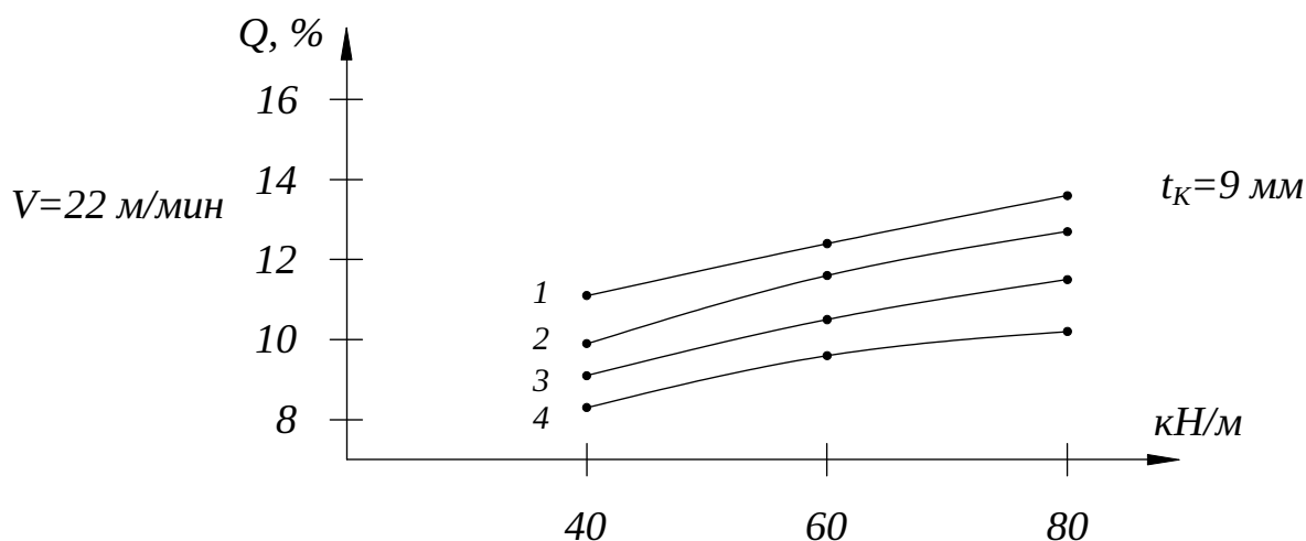
Рисунок 5. График удаленной влаги из кожевенного полуфабриката от сочетания пар отжимных валов, давления прижима P=40; 60; 80 кН/м и скорости пропускa V=22 м/мин
