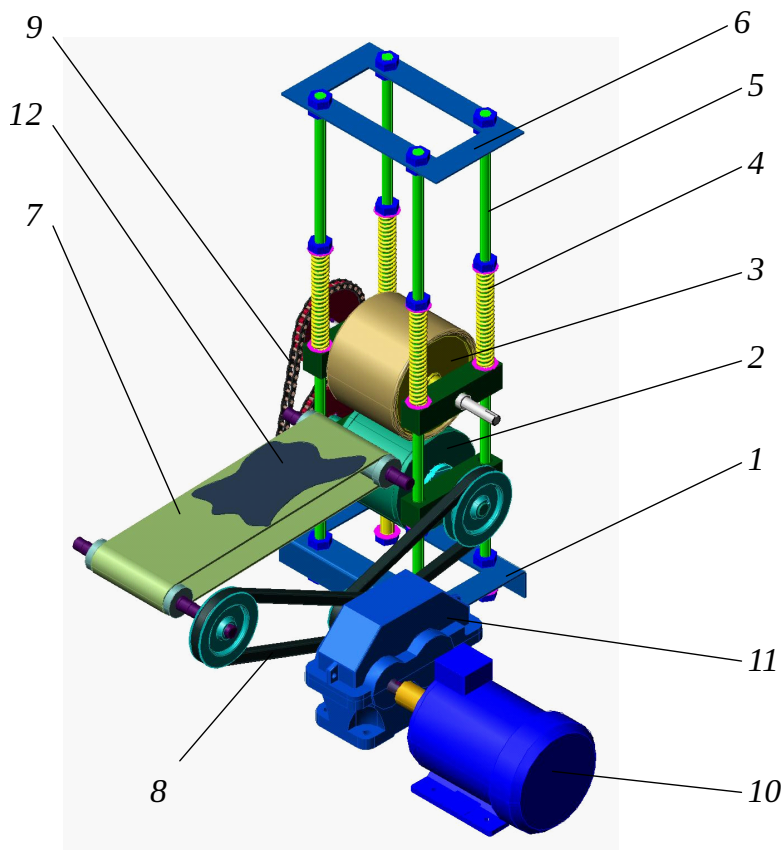
Рисунок 1. Модель экспериментального валкового стенда
