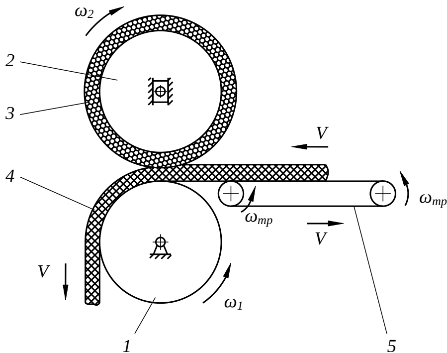
Рисунок 2. Схема работы валковой пары отжимной машины. 1 – металлокерамический вал; 2 – стальной вал; 3 – маншионовая покрывка; 4 – коженый полуфабрикат; 5 – транспортер
