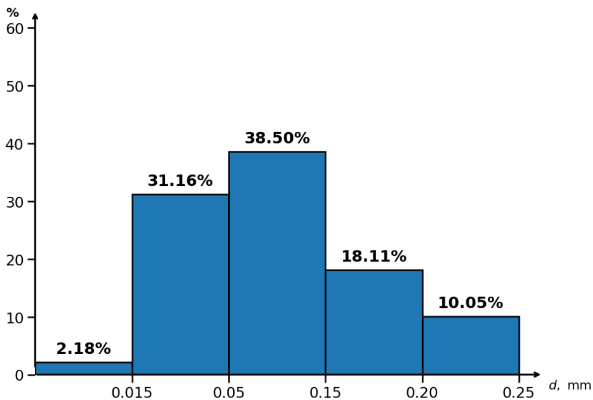
Рисунок 2. Распределение частиц кварцевого песка по размерам зерен.
