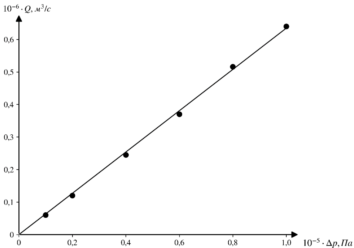
Рисунок 3. Зависимость объемного расхода воды от перепада давления.
