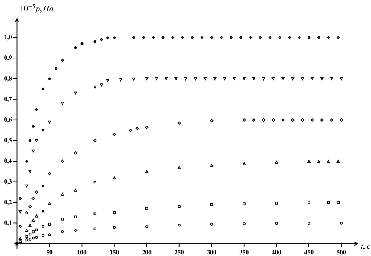
Рисунок 4. КВД при 10^{-5} p_0 = 0, 1 ( \circ ), 0, 2 ( \square ), 0, 4 ( \triangle ), 0, 6 ( \diamond ), 0, 8 ( \nabla ), 1, 0 ( + ), Па.
