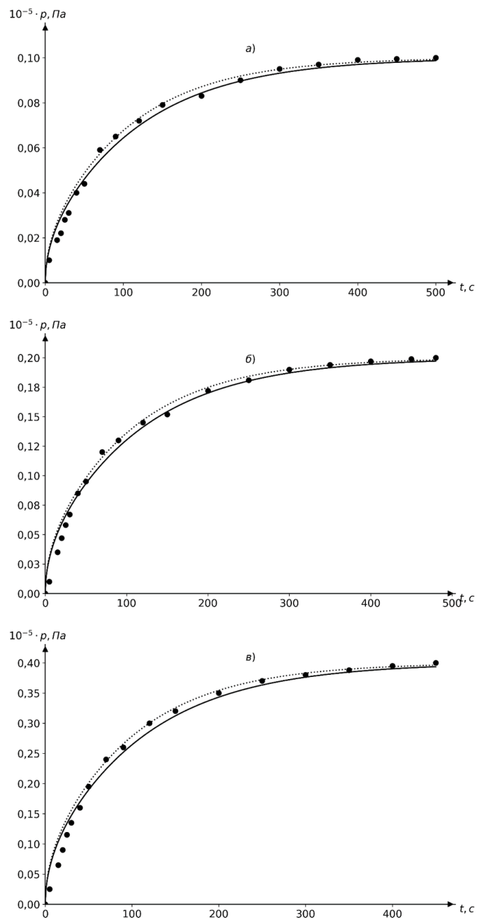
Рисунок 5. Экспериментальные данные (•) и расчетные кривые p(t, L) по данным табл. 1 и 2 при 10^{-5} p_0 = 0,1 (а), 0,2 (б), 0,4 (в), Па.
