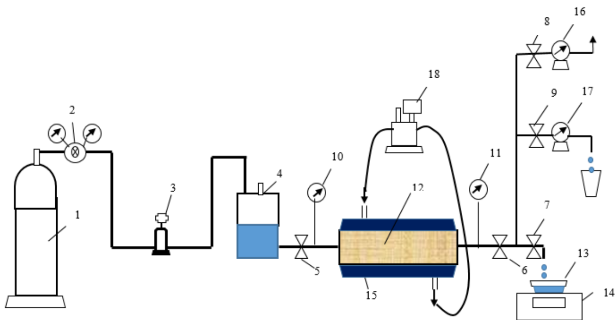
Рисунок 1. Установка по определению фильтрационных характеристик модели пористой среды. 1 – баллон высокого давления для воздуха, 2 – редуктор давления, 3 – стабилизатор давления, 4- емкость для жидкости, 5,6,7,8,9 – вентили, 10,11 – образцовые манометры, 12 – модель пористой среды, 13 – измерительная посуда, 14 – электронные весы, 15 – рубашка для циркуляции теплоагента, 16 – газовый счетчик, 17 – расходомер для жидкости, 18 – термостат.
