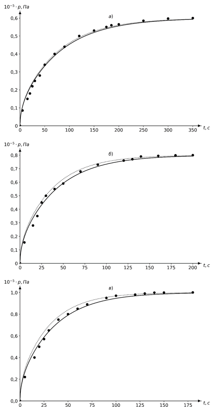
Рисунок 6. Экспериментальные данные (•) и расчетные кривые p(t, L) по данным табл. 1 и 2 при 10^{-5} p_0 = 0,6 (а), 0,8 (б), 1,0 (в), Па .
